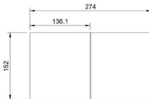
VISTA SUPERIOR
