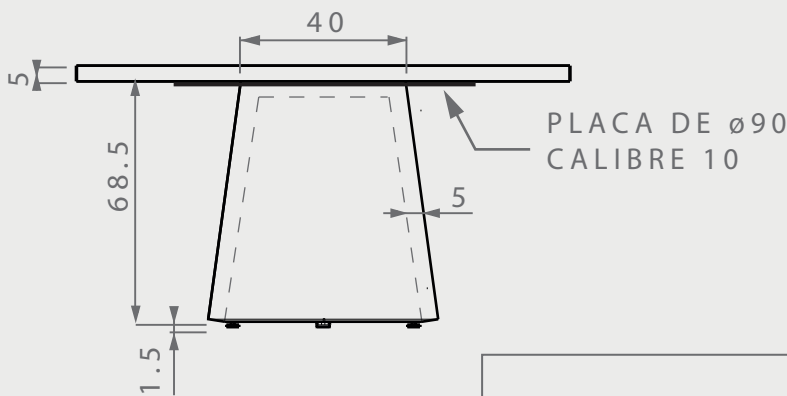
VISTA LATERAL
