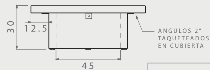
VISTA LATERAL
