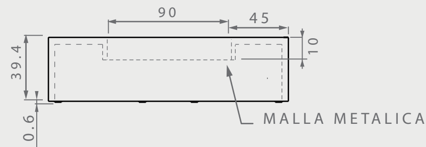
VISTA LATERAL
