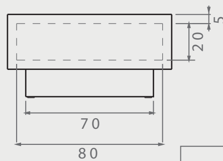
VISTA LATERAL
