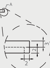
VISTA DETALLE:A
